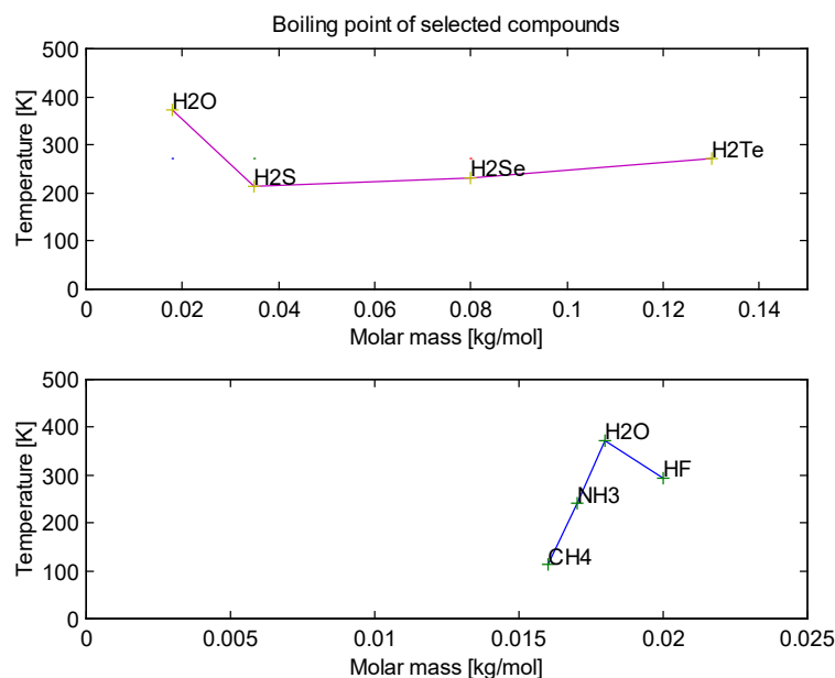
Fig. 14. Anomalia del punto de ebullición normal del agua frente al de otros hidruros del grupo VI y a otros compuesto de hidrógeno del periodo 2 del sistema periódico de los elementos.
